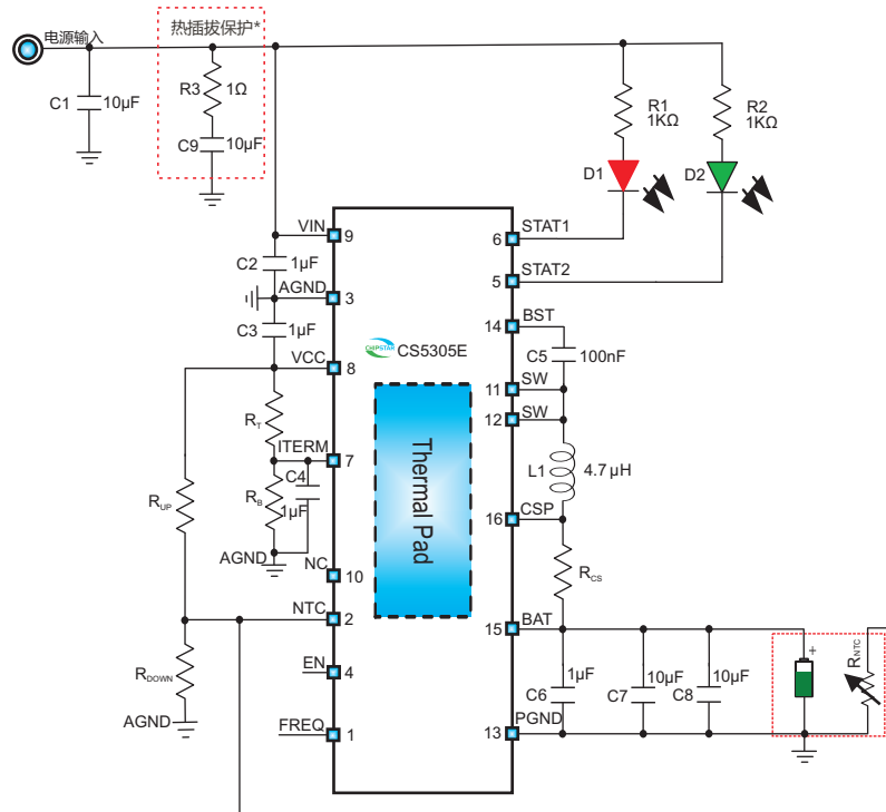
CS5305E应用电路图
