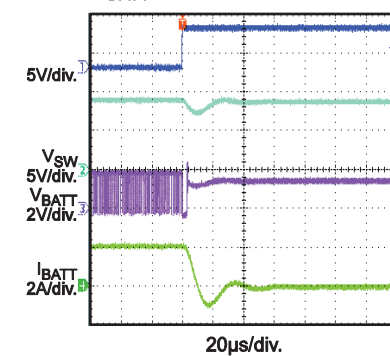
En Off V_{BATT} = 3.6V
